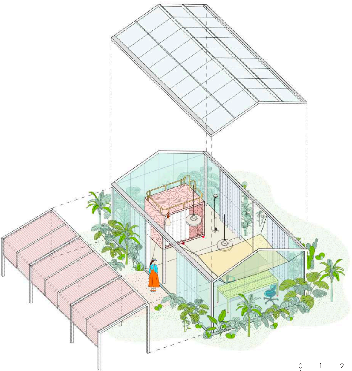
/ VISTA AXONOMÉTRICA
