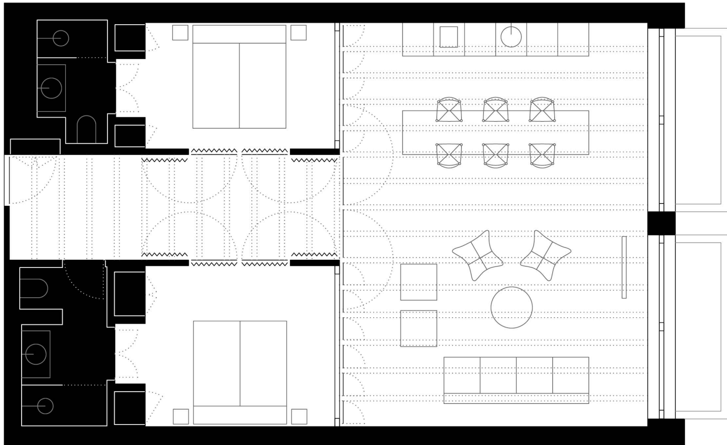
Planta de proyecto.
